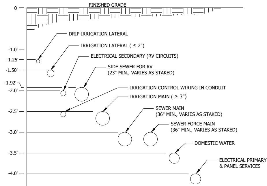
UTILITY DEPTH DIAGRAM N.T.S.
